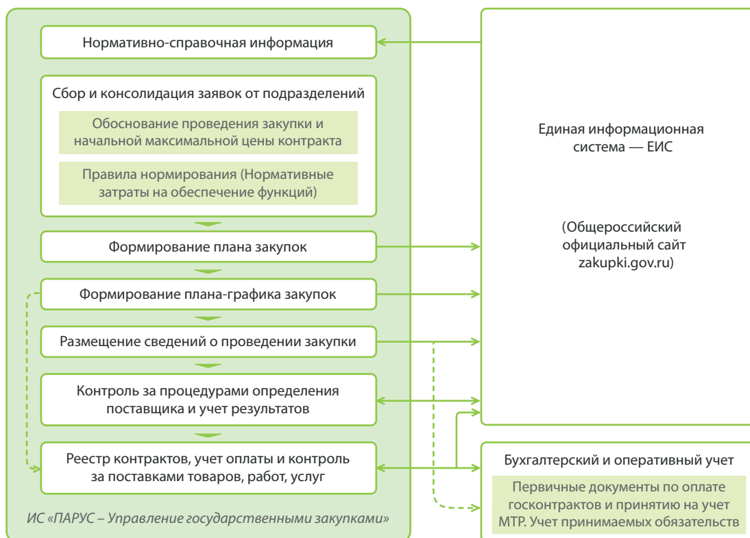
Рис. 1. Функциональные возможности системы
