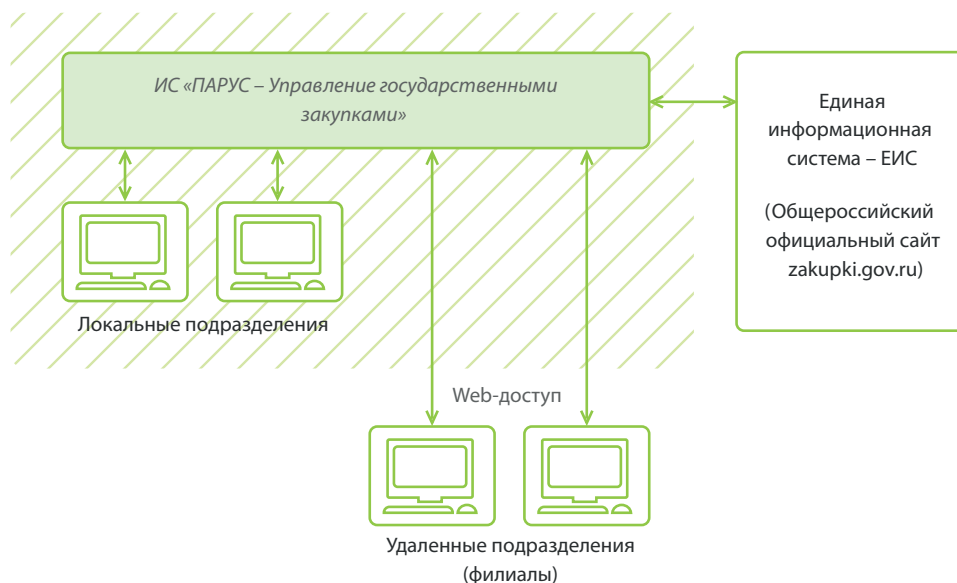
Рис. 2. Архитектура решения «ПАРУС – Управление государственными закупками»
